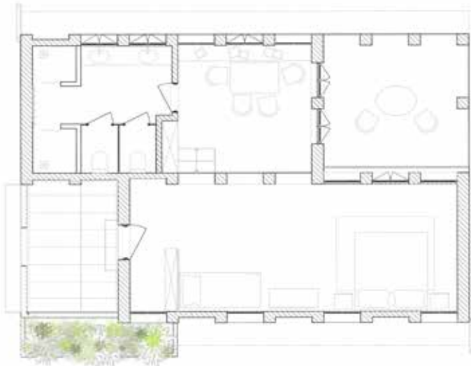
Grundriss Gästehaus floor plan guest house
