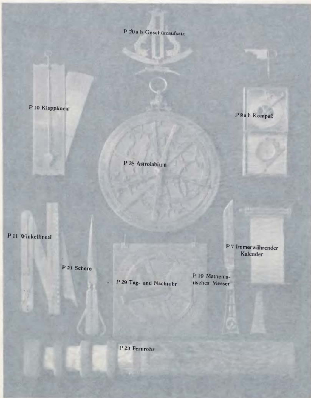
Tafel XXIV. Instrumente aus vergoldetem Messing u. a. (S. 39 ff.)
